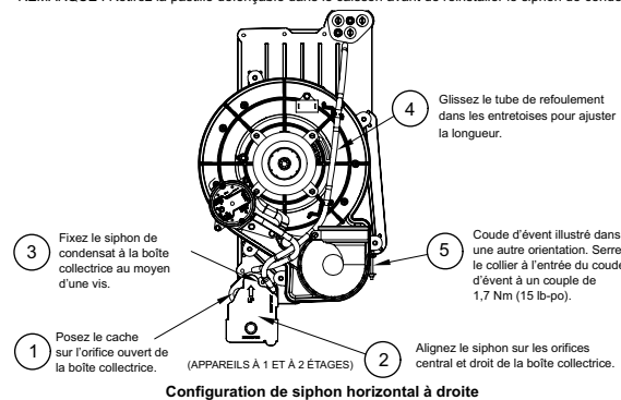
Figure 10 – Configurations de siphon à tirage horizontal à droite (l'apparence peut varier)
