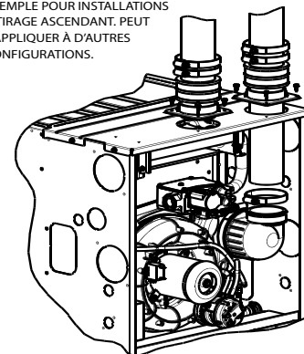
Figure 45 – Exemple de raccordement de tuyau d'admission d'air pour des systèmes de ventilation en polypropylène
