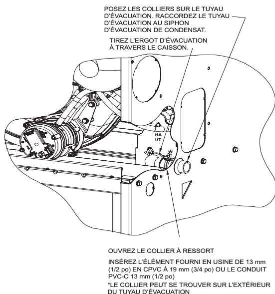
INSTALLATION DU TUYAU D'ÉVACUATION À DROITE
