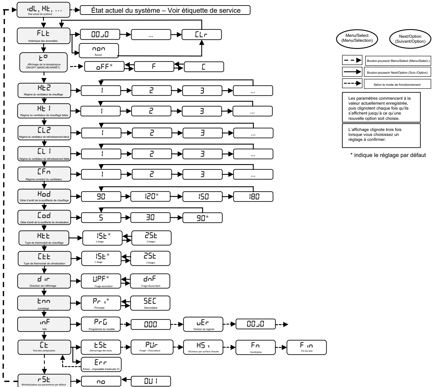
Figure 59 – Organigramme de l'écran à trois chiffres
