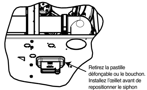
Figure 18 – Œillet de siphon d'évacuation horizontal
