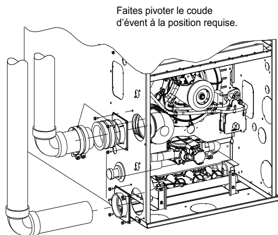
CONFIGURATION À GAUCHE À TIRAGE DESCENDANT
