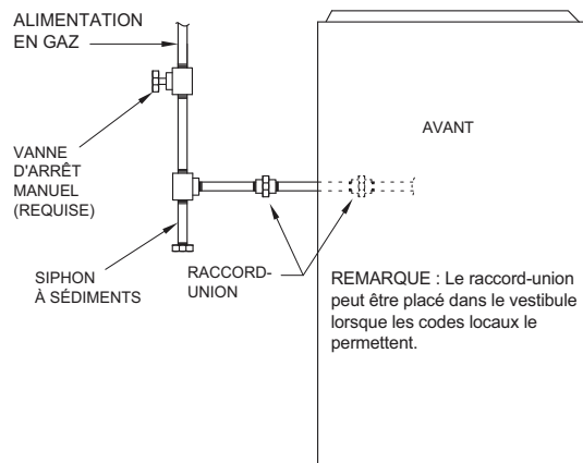
Figure 32 – Disposition type de la tuyauterie de gaz
