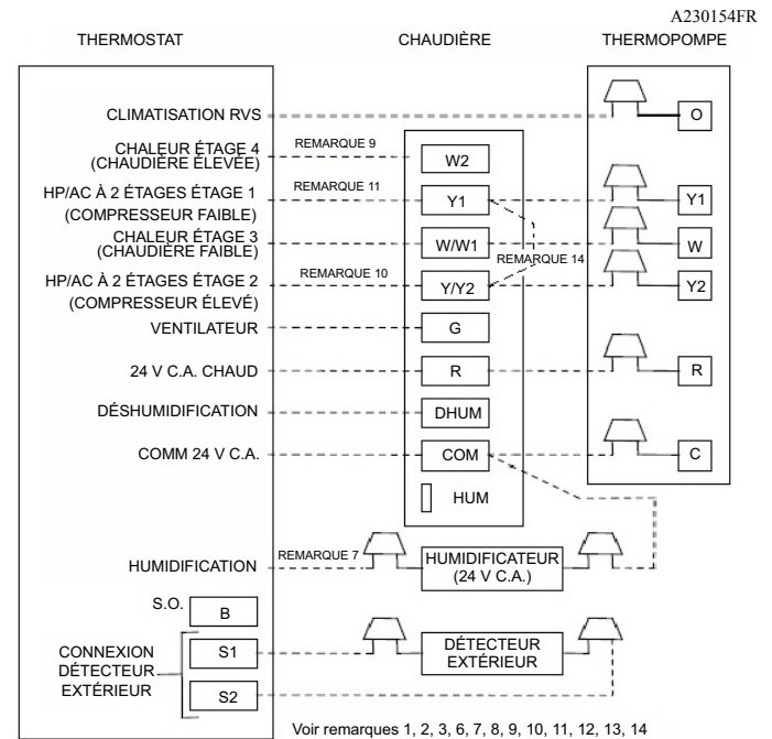
Chaudière à deux étages avec thermopompe
