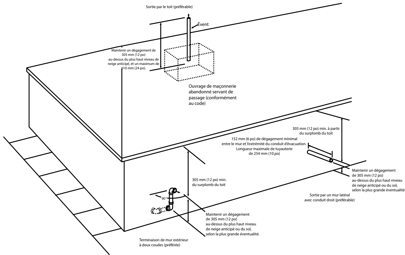
Figure 41 – Sortie d’évent pour système à évacuation indirecte et à air de combustion ventilé
