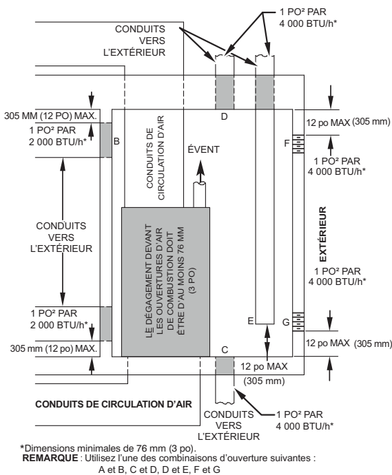
Figure 6 – Air de combustion, de ventilation et de dilution vers l'extérieur
