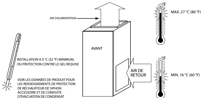
Figure 3 – Protection contre le gel et température de l'air de retour
