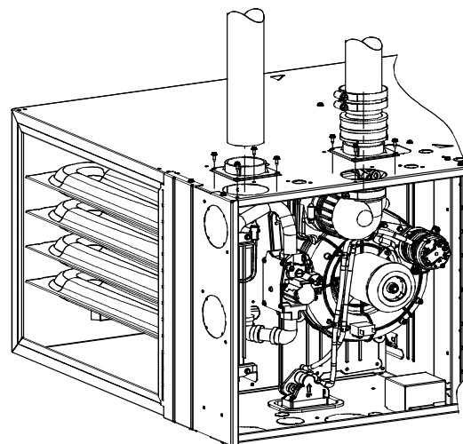
A11327A CONFIGURATION HORIZONTALE À GAUCHE À ÉVACUATION VERTICALE
