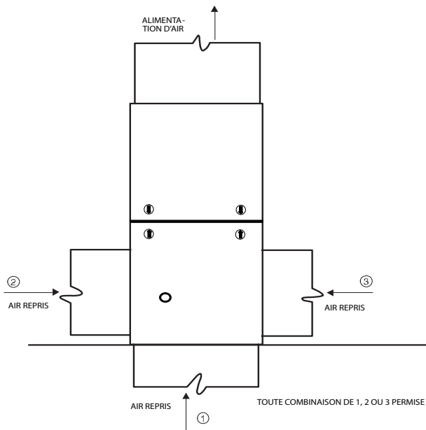
Figure 21 – Configurations et restrictions des conduits d'air de retour en tirage ascendant
