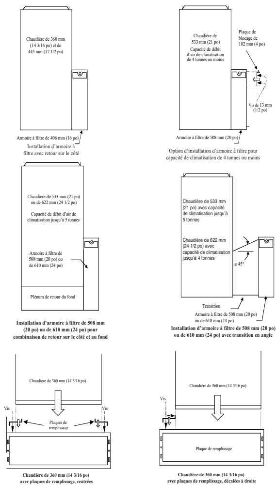
Figure 27 – Armoire de filtration en option
