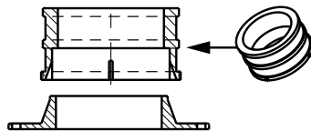
Adaptateur et raccord d'évent
