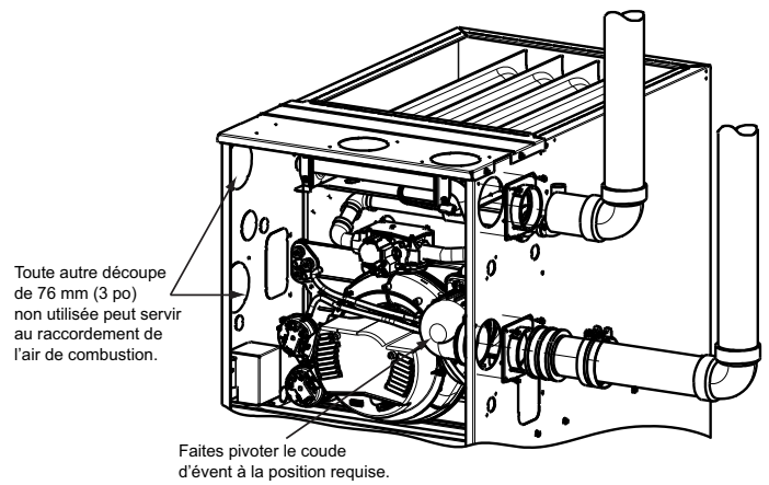
CONFIGURATION À DROITE À TIRAGE ASCENDANT
