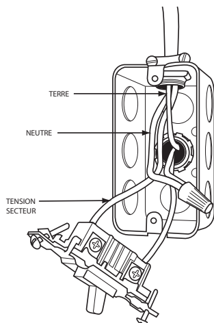
Figure 36 – Coffret électrique externe fourni sur place fixé au caisson de la chaudière
