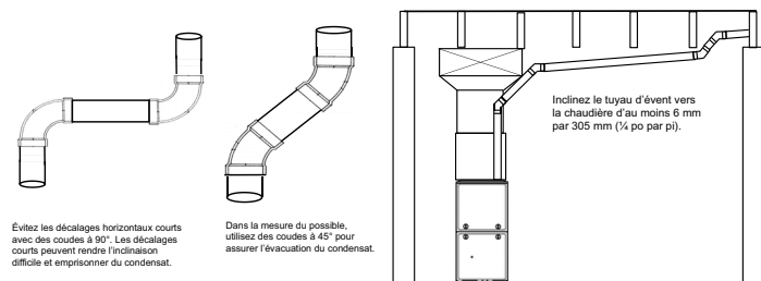
Figure 52 – Raccordement d'évent près de la chaudière
