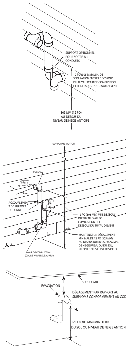
Figure 49 – Sortie d'évent pour l'Alberta et la Saskatchewan
