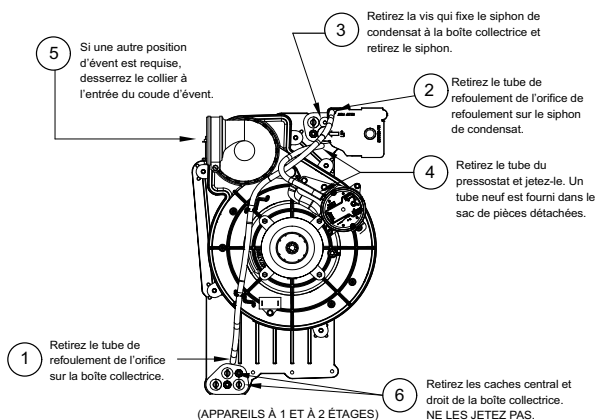
Figure 10 – Configurations de siphon à tirage horizontal à droite (l'apparence peut varier)
