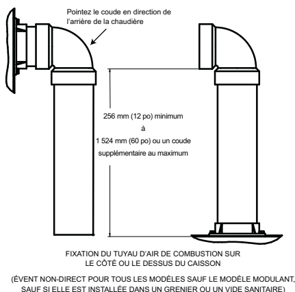
Figure 47 – Fixation du tuyau d'air de combustion
