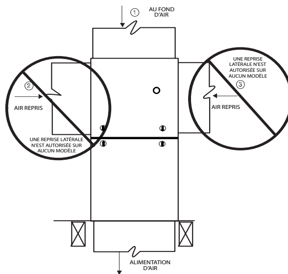
Figure 22 – Configurations et restrictions des conduits de retour en tirage descendant
