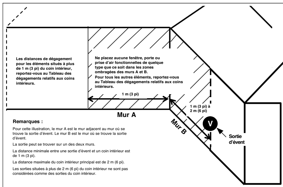
Figure 44 – Sorties dans les coins intérieurs
