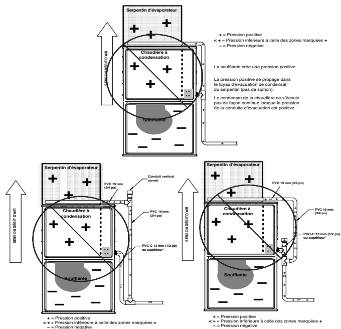
Figure 13 – Exemple de fixation du tuyau d'évacuation sur place (non autorisée)
