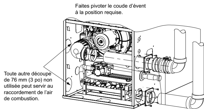
A230013FR CONFIGURATION À DROITE À TIRAGE DESCENDANT
