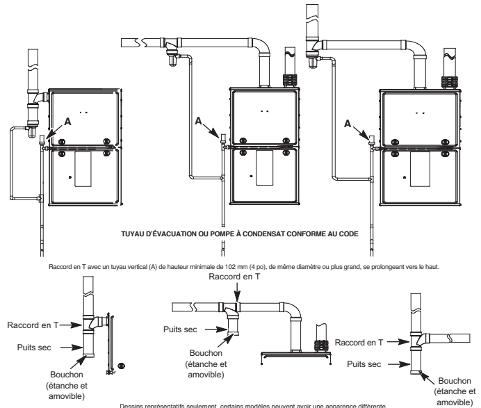
Figure 51 – Pot de condensation de tuyau d'entrée d'air de combustion recommandé
