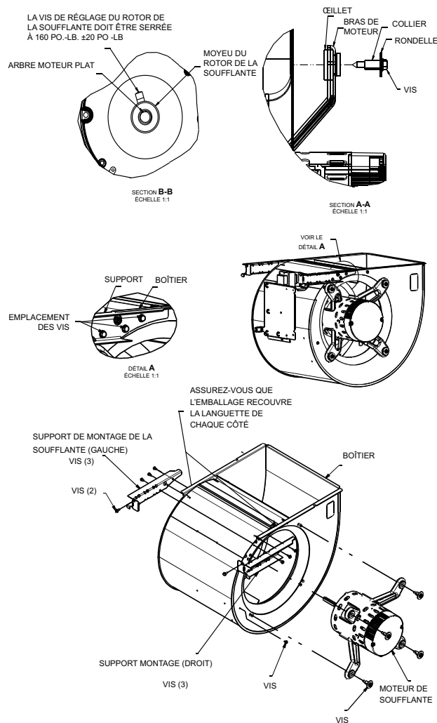
Figure 67 – Ensemble de soufflante sur 100V21--22 A190407FR
