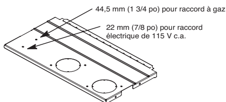
Figure 31 – Autre entrée de gaz et d'électricité
