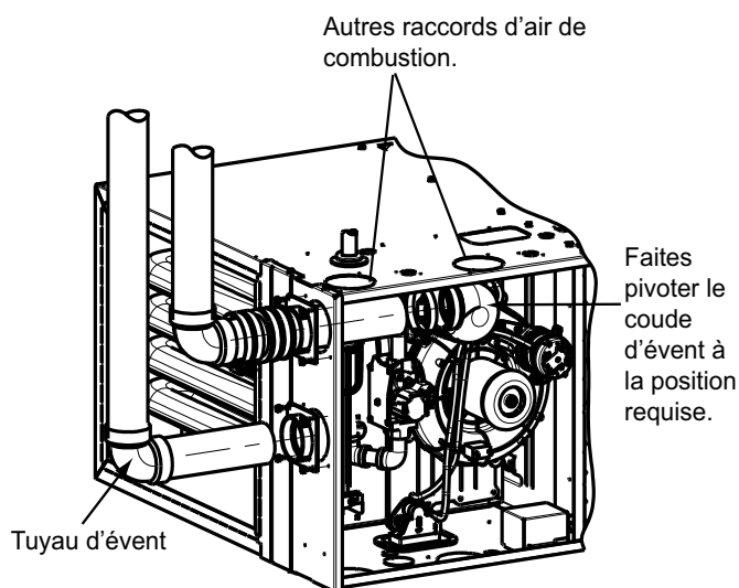
A11328AFR CONFIGURATION HORIZONTALE À GAUCHE ET À ÉVENT À GAUCHE
