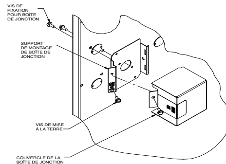
Figure 35 – Installation d'une boîte de jonction (le cas échéant)
