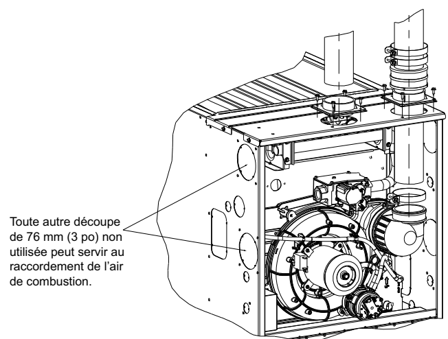
ÉVÉNEMENT VERTICAL À TIRAGE ASCENDANT
