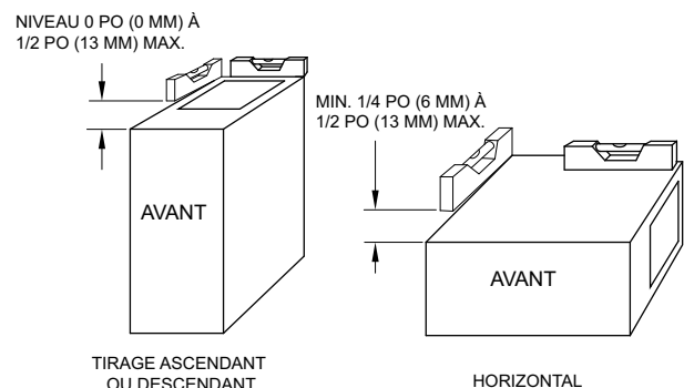
Figure 19 – Exigences d'inclinaison de la chaudière
