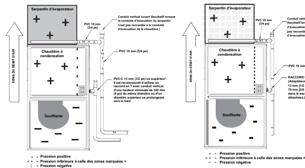
Figure 12 – Exemple de fixation du tuyau d'évacuation sur place
