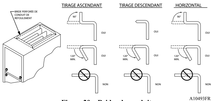
Figure 20 – Brides de conduit
