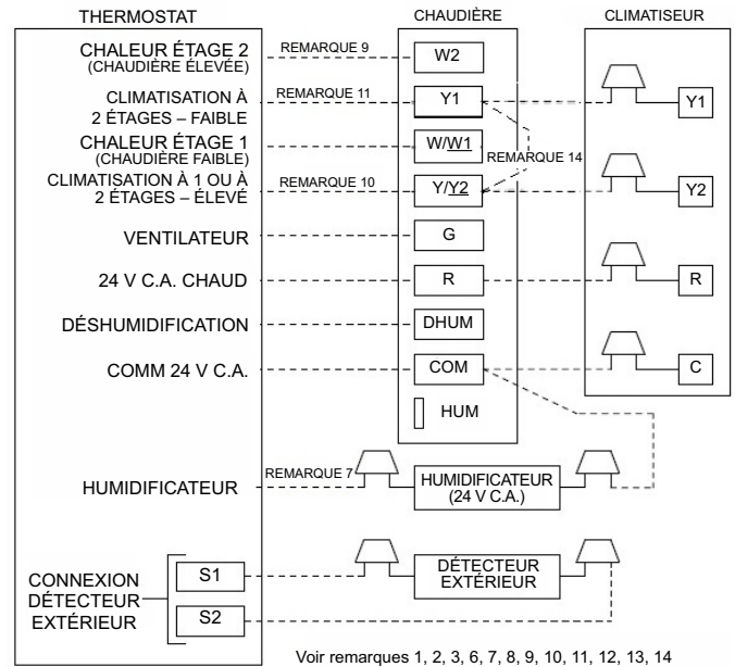
Chaudière à deux étages avec climatiseur
