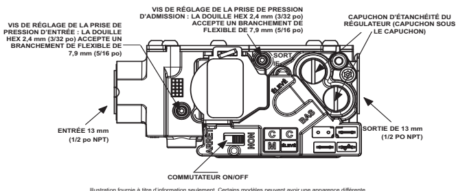
Figure 64 – Soupape de gaz avec orifices de pression
