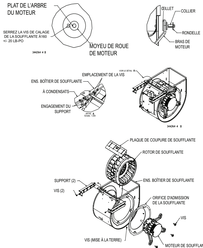
Figure 66 – Ensemble de soufflante
