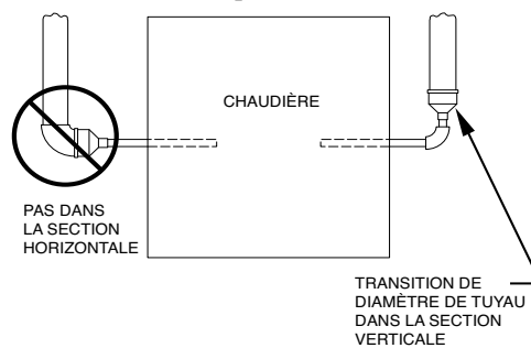
Figure 50 – Emplacement du changement de diamètre de tuyau d'évent et d'air de combustion et configuration du coude
