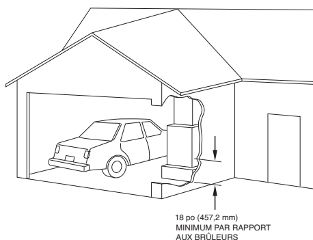
Figure 5 – Installation dans un garage
