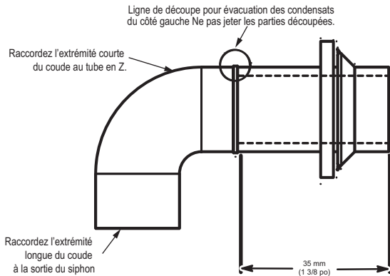
Figure 17 – Modification du coude d'évacuation en caoutchouc
