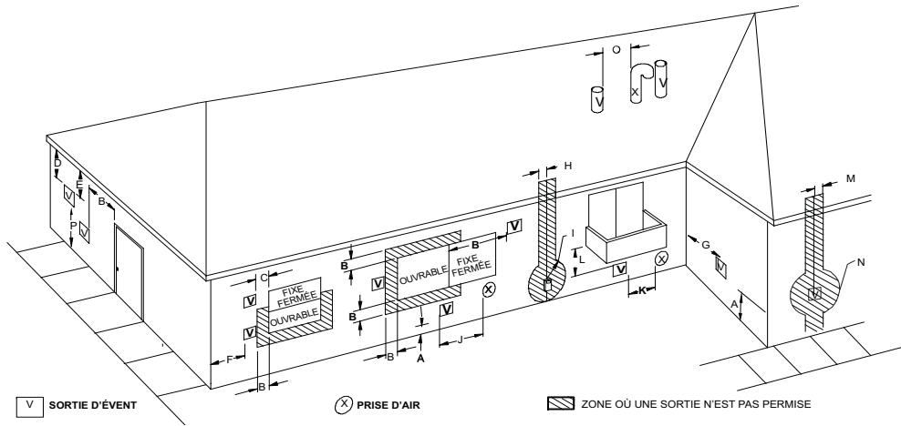
Figure 42 – Dégagement de sortie d’évacuation directe
