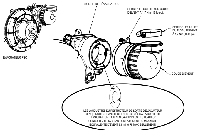
Figure 53 – Coude d'évent de l'évacuateur
