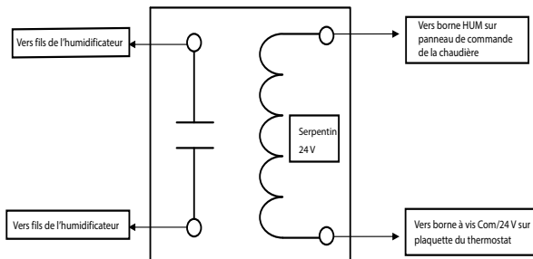
Figure 37 – Relais d'isolation pour humidificateurs, fourni sur place, avec bloc d'alimentation interne
