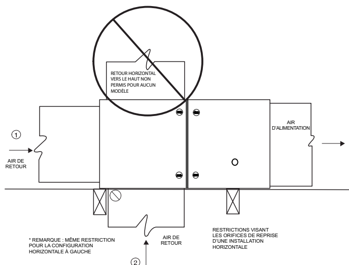
Figure 23 – Configurations et restrictions des conduits de retour à l'horizontale
