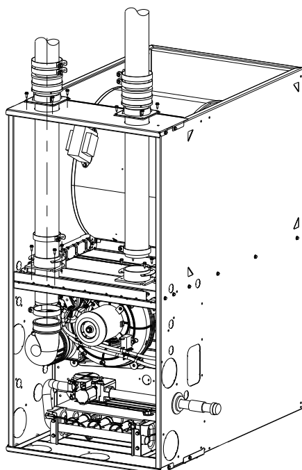
A230013FR CONFIGURATION À DROITE À TIRAGE DESCENDANT
