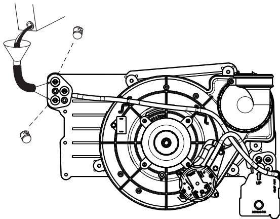
CONFIGURATION DE SIPHON À TIRAGE ASCENDANT APPAREILS A 1 ET A 2 ÉTAGES
