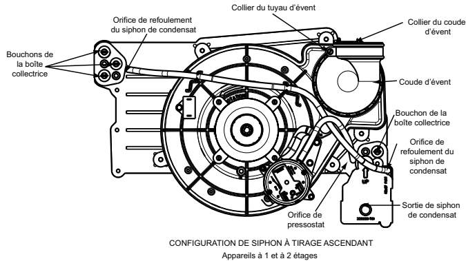
Figure 8 – Configurations de siphon à tirage ascendant (l'apparence peut varier)
