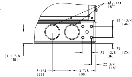
DETAIL C TYP 4 PLCS
