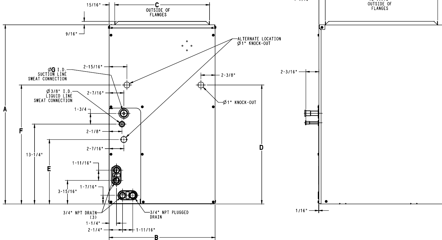
Fig. 2 – Dimensions (English)
