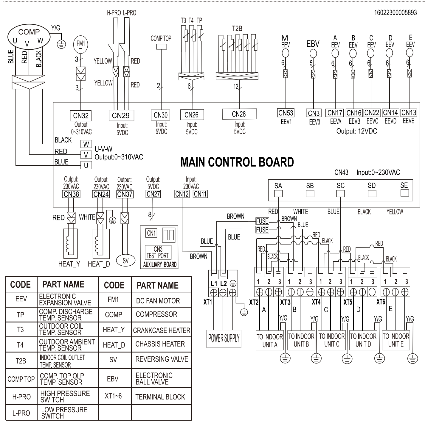
Fig. 16 — Wiring Diagram 30K/36K
